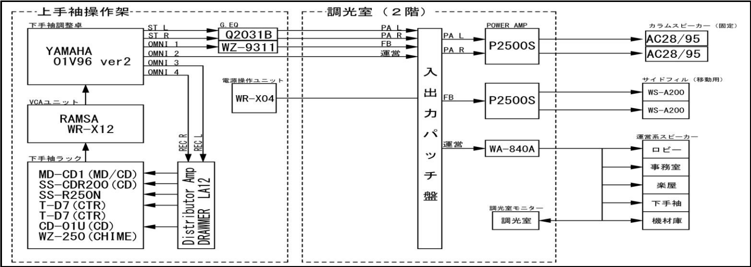
音響システム系統図
